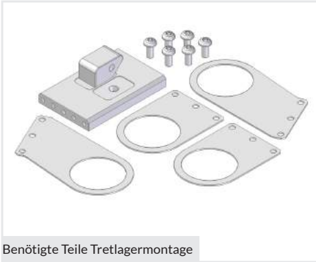
Benötigte Teile Tretlagermontage
