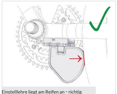
Einstelllehre liegt am Reifen an - richtig
