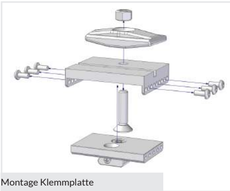
Benötigte Teile Montage Klemmplatte
