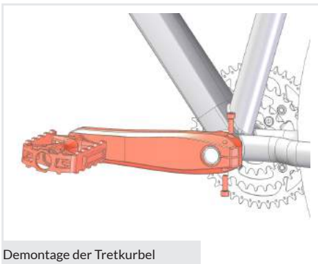
Demontage der Tretkurbel
